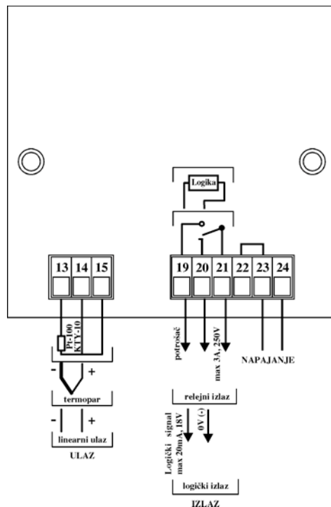
Slika 1.1. Prikaz povezivanja sa zadnje strane uređaja
