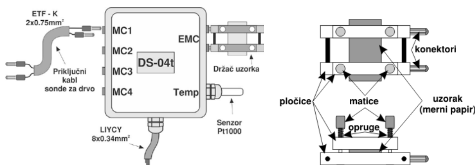
Slika 2.5. Povezivanje mernih elemenata na kutiju DS-04t i držač uzorka
