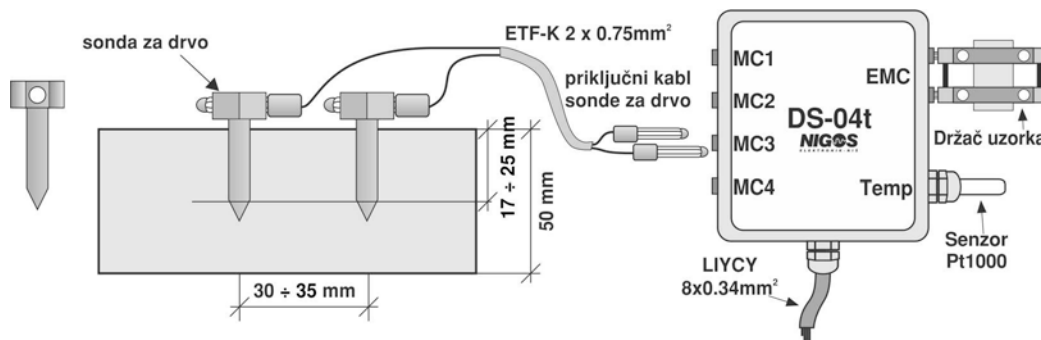
Slika 2.6. Povezivanje sondi za drvo
