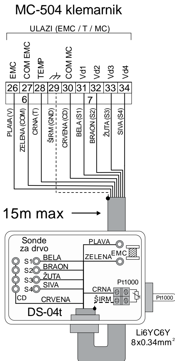
Slika 2.4. Šema povezivanja merne kutije DS-04t i MC-504
