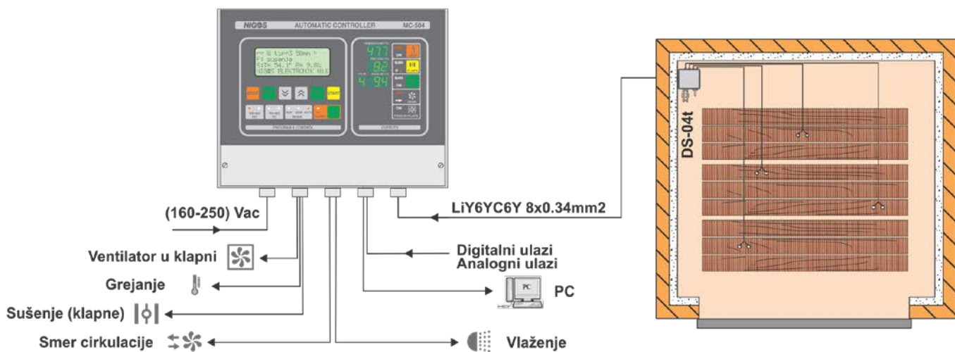
Slika 2.1. Blok šema povezivanja automata MC-504 u sistemu sa 1 mernim mestom za temperaturu i ravnotežnu vlagu i 4 mernih mesta za vlagu u drvetu
