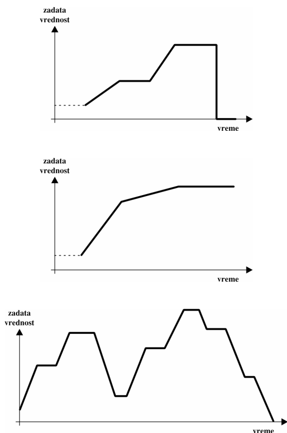
Slika 4.1 Primeri programa
