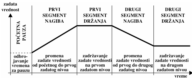
Slika 4.3 Segmenti programa
