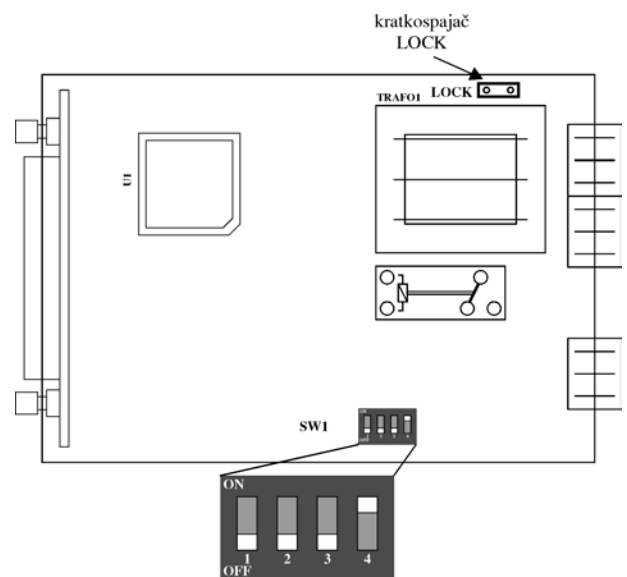
Slika 3.1. Položaj kratkospajča LOCK i DIP SWITCH - a SW1 na donjoj ploči uređaja
