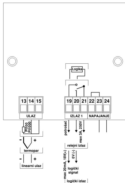
Slika 1.1. Prikaz povezivanja sa zadnje strane uređaja
